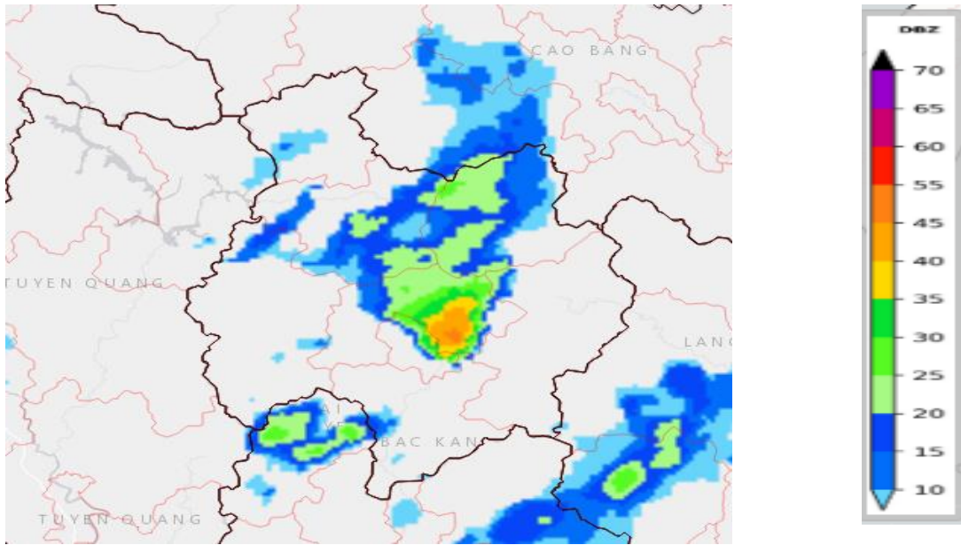
Ảnh ra đa tại Bắc Kạn lúc 16h30' ngày 19/9
